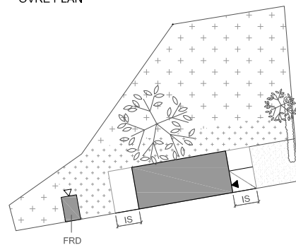
ÖVRE PLAN
