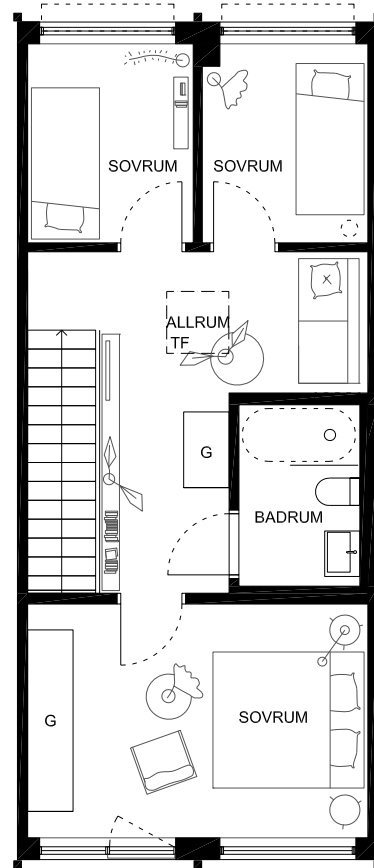
ÖVRE PLAN
