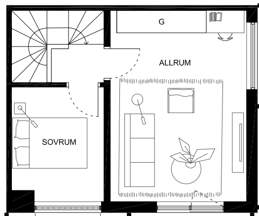
ÖVRE PLAN
